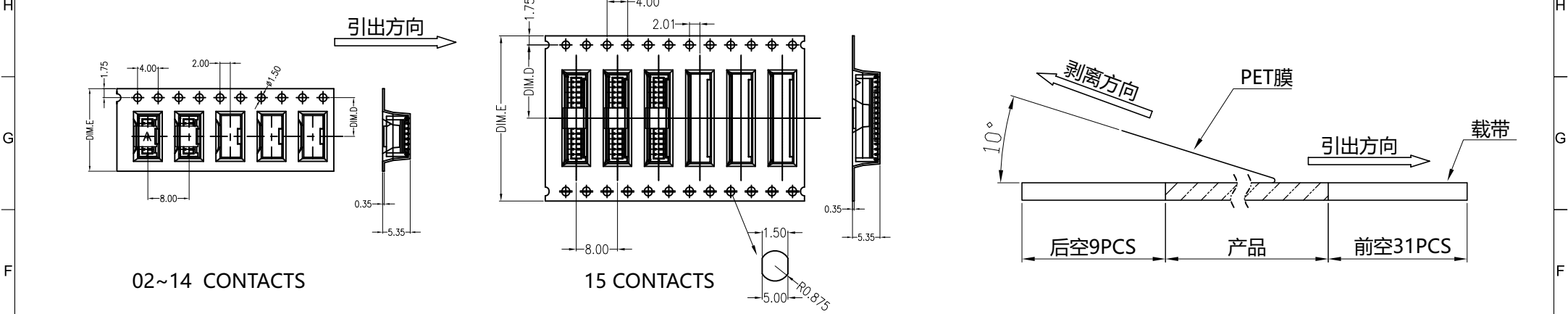
(PET膜剥离示意图)
