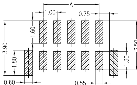
PCB Layout 线路板印刷示意图
