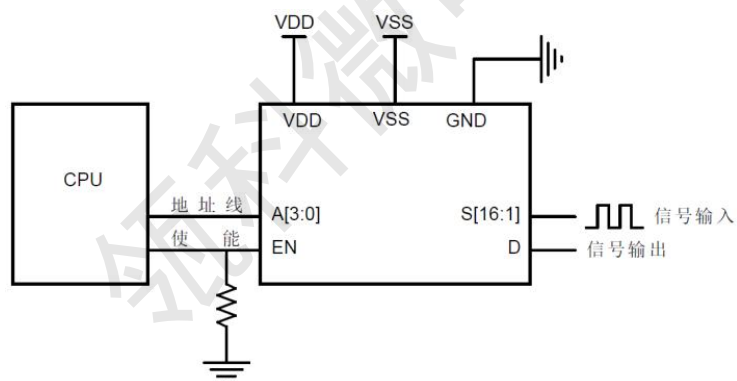
图 11 典型应用
