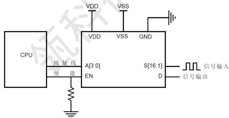
图 1 典型应用图
