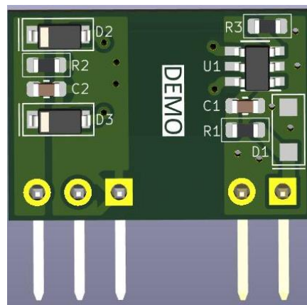
图 3.3 PCB 版图背面
