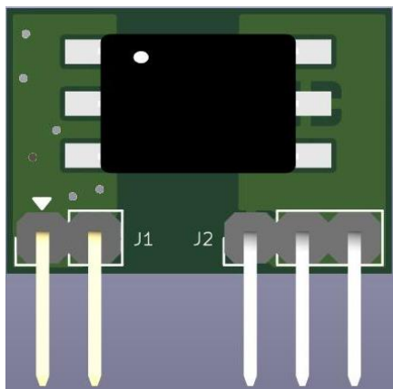
图 3.2 PCB 版图正面
