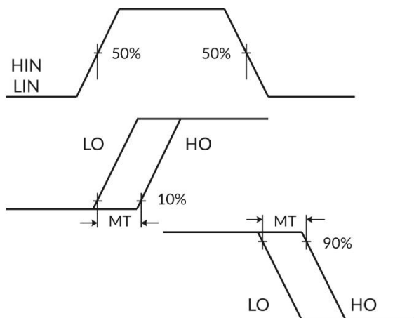
图 3. 延迟匹配波形图
