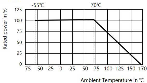
功率曲线
