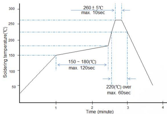
回流焊曲线图
