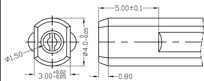
轴心部尺寸详图 2:1
