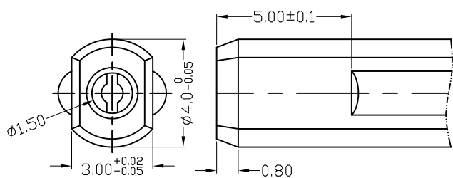
轴心部尺寸详图
