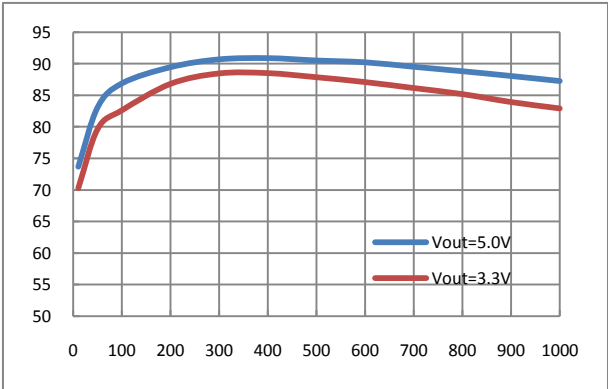
Efficiency@VIN=12V
