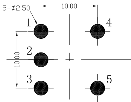
底部铜箔接触位置
