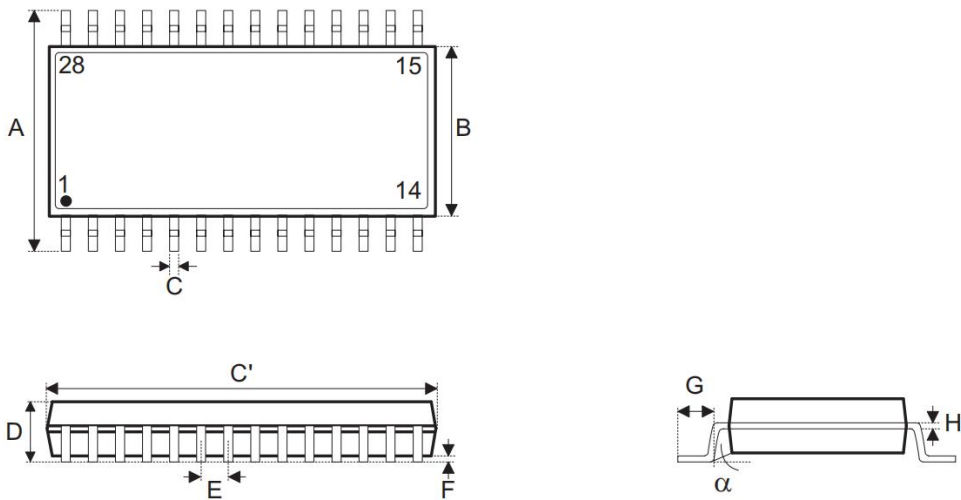
SOP28（300mil）外形图与封装尺寸
