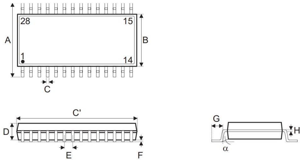
SSOP28（150mil）外形图与封装尺寸
