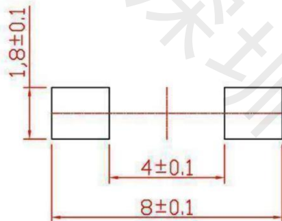
PCB. 焊接图
