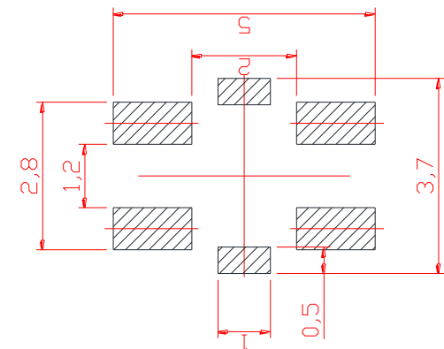
PCB. 焊接图
