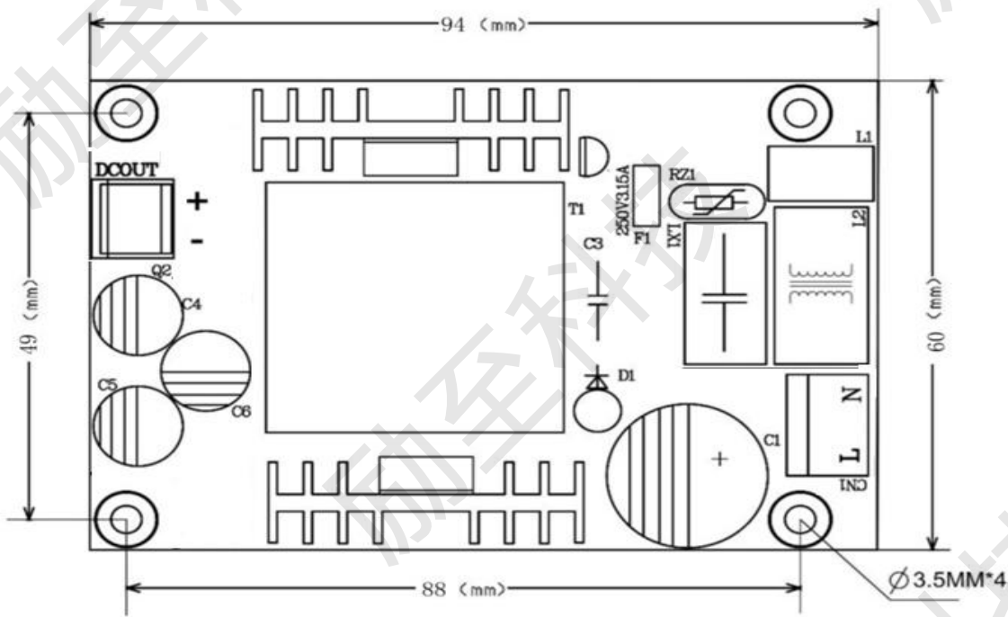
机构尺寸图:
