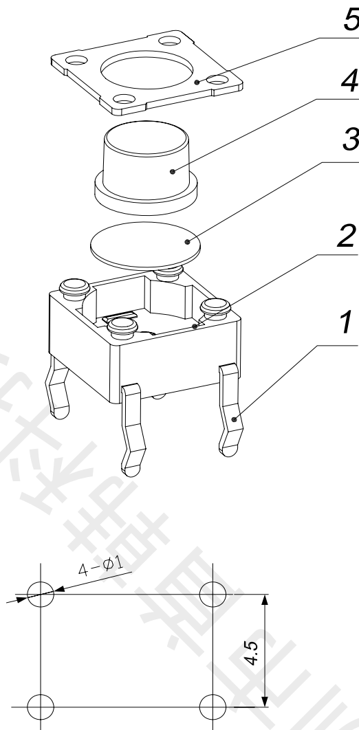
印制线路板 Recommended P.C.B layout
