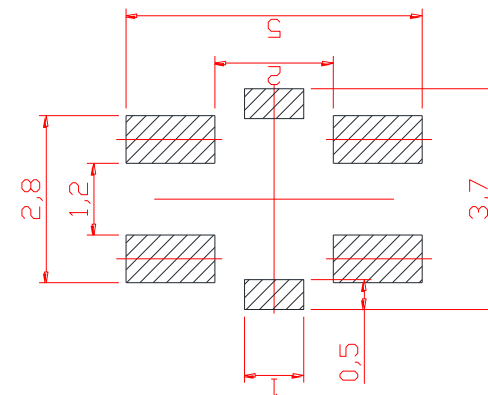
PCB. 焊接图
