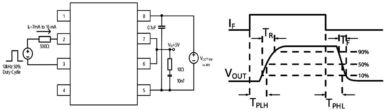
Fig.18 T_{PHL} 、 T_{PLH} 、 T_R 、 T_F Test Circuit
