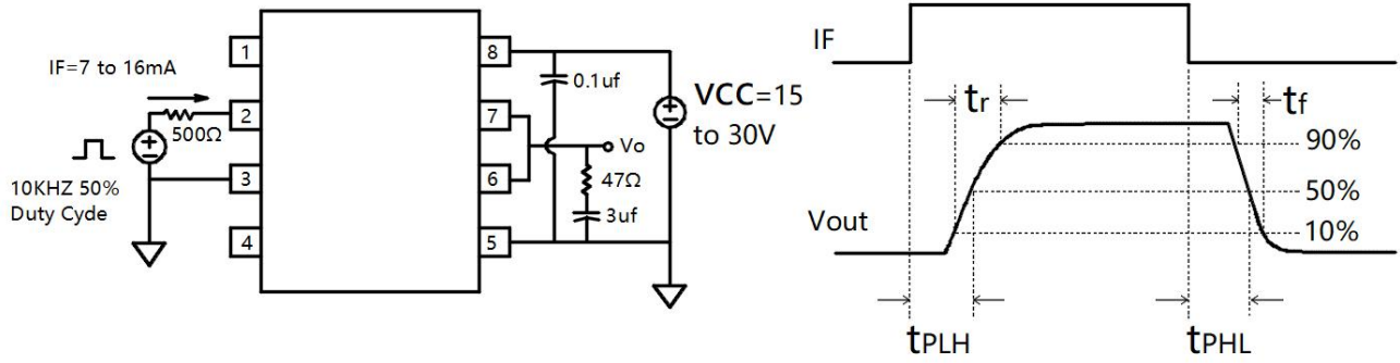
Fig.18 T PHL 、T PLH 、T R 、T F Test Circuit
