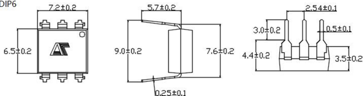
DIP6
