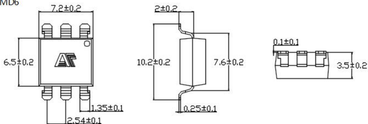
SMD6
