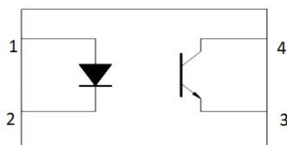
引脚配置 Pin Configuration
