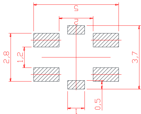
PCB. 焊接图
