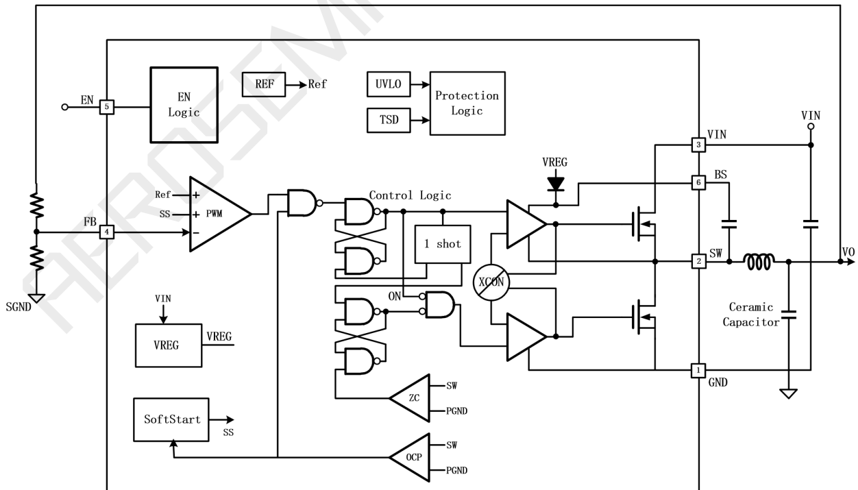
图 2. MT2496 内部框图
