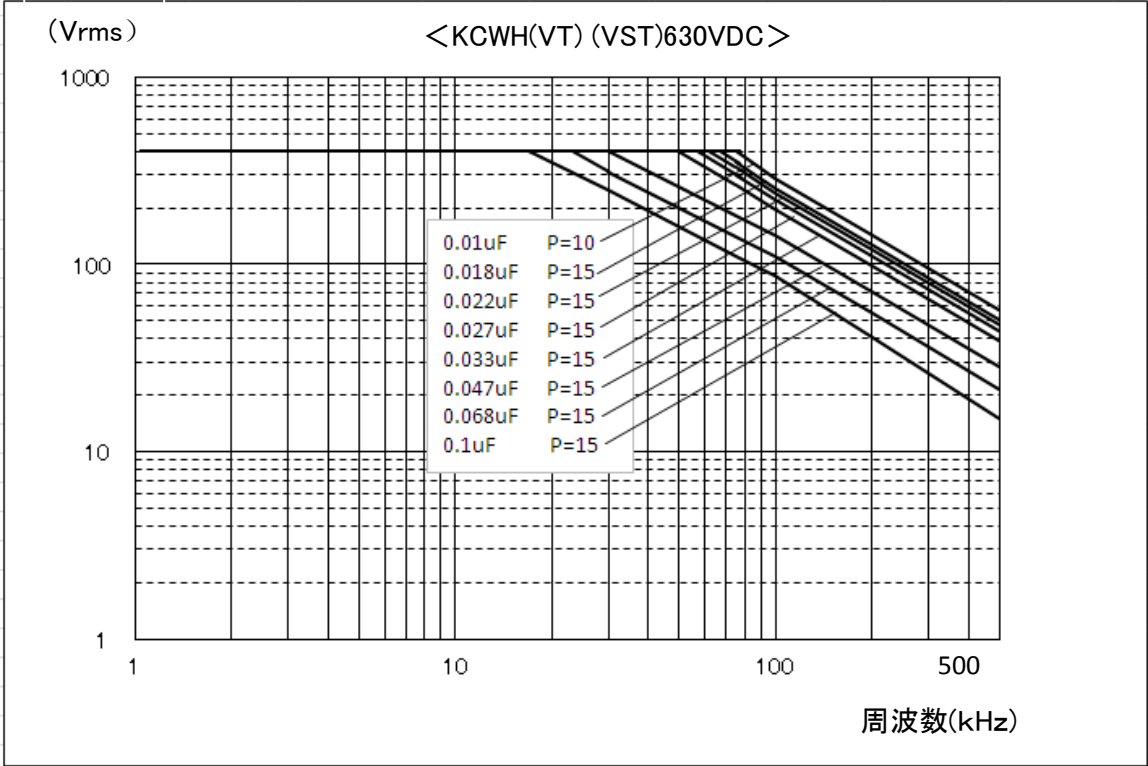
【Fig.6 图-6 1000VDC】 (75℃—100℃ 每 1℃ 轻减 1.35%。)
