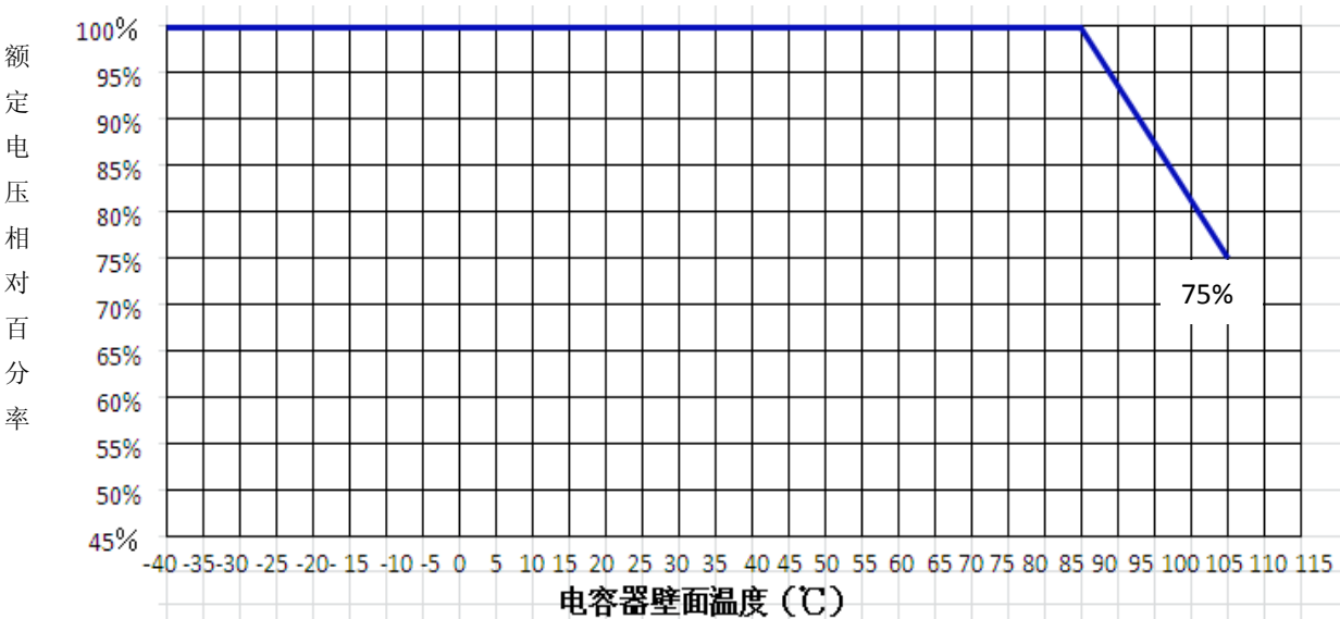
图-2 使用温度相对容许电流, 容许脉冲电流值的衰减曲线
