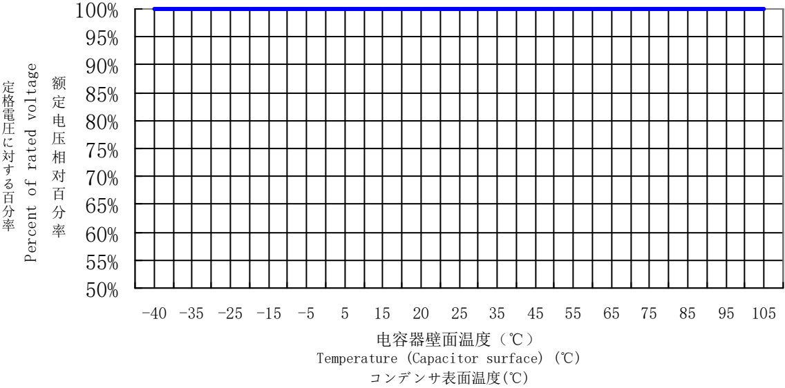
图-2 使用温度相对容许电流，容许脉冲电流值的衰减曲线 FIG. 2 CURRENT DERATING VS TEMPERATURE 図-2 使用温度に対する許容電流，許容パルス電流値の軽減曲線
