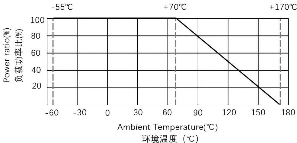
功率衰减曲线图 / Derating Curve
