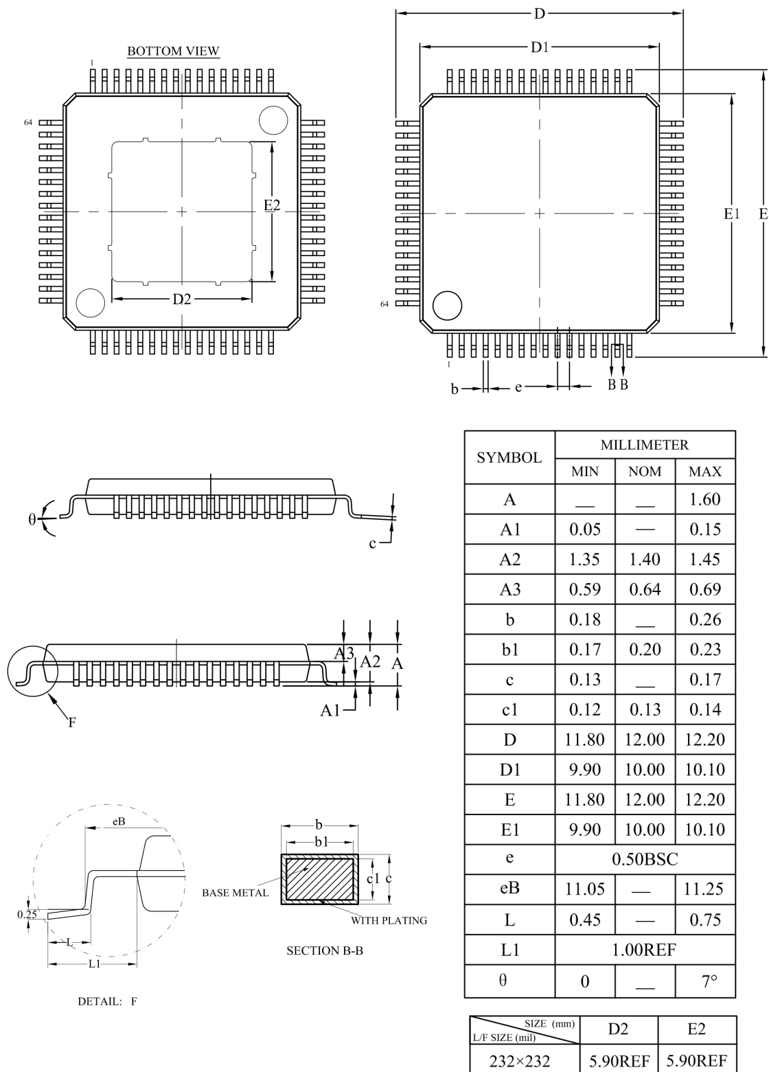
图 29: 64eLQFP 封装尺寸图
