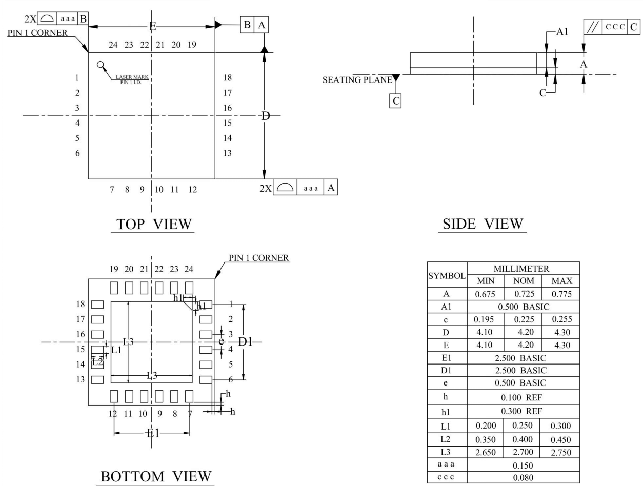
图 12 封装外形
