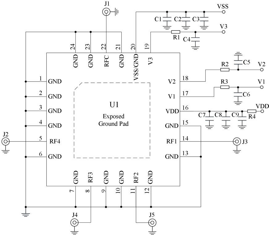
图 11 应用电路
