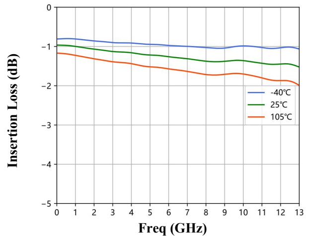
图6 三温, RF2导通插入损耗
