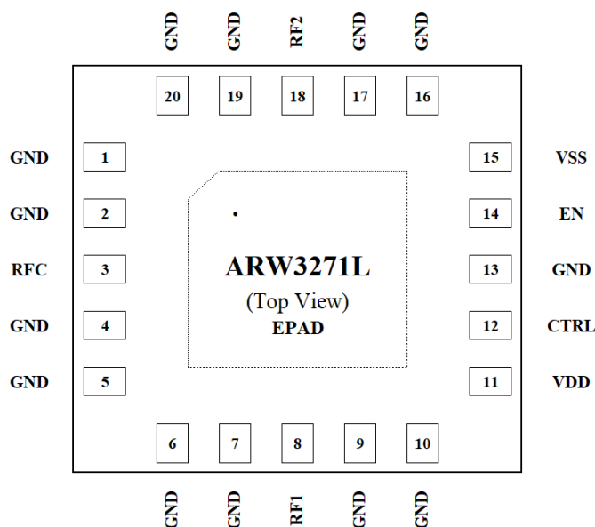
图 2 引脚说明
