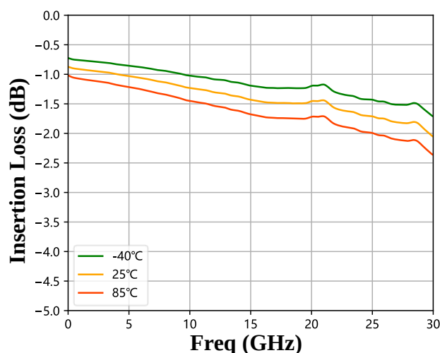
图7 三温，RFC to RF1/RF2插损
