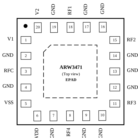
图 2 引脚说明
