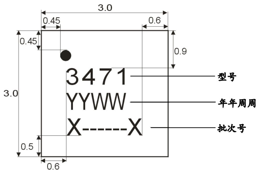
图 14 器件标识
