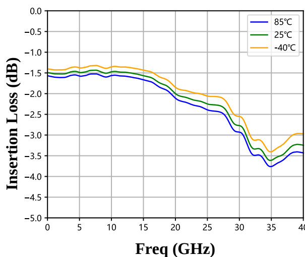
图10 三温，RFC to RF2插损
