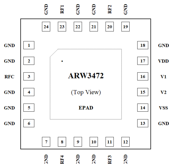
图 2 引脚说明
