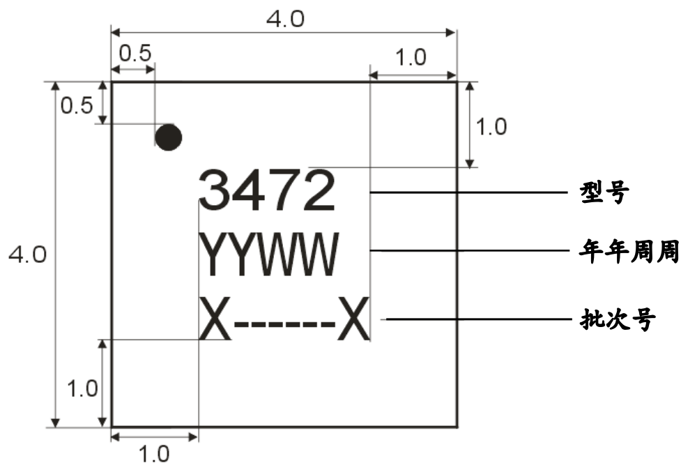
图 17 器件标识
