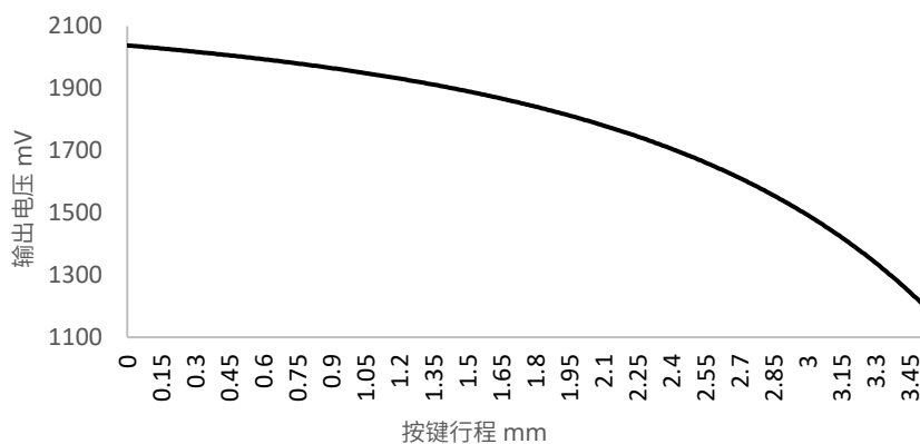
图 6. 按键行程与输出电压
