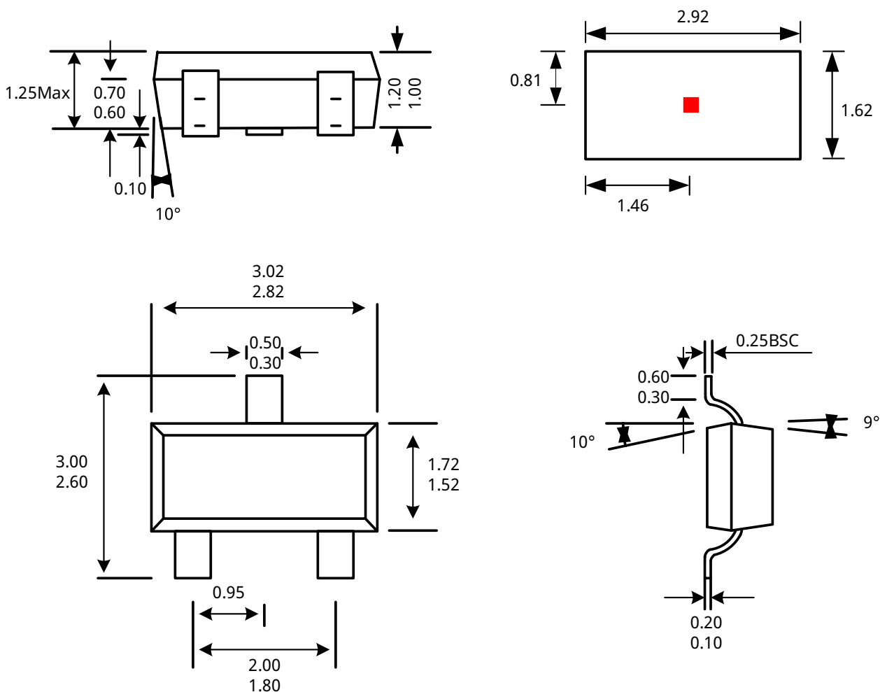
3-脚 SOT23-3L 封装
