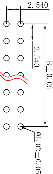
P.C.B LAYOUT
