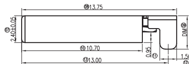
外壳DIP脚长度 (DIM:A=3.00)
