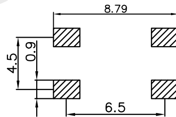
安装参考图
