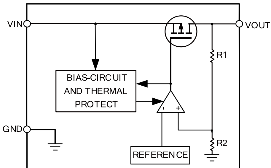
图 1. 功能框图
