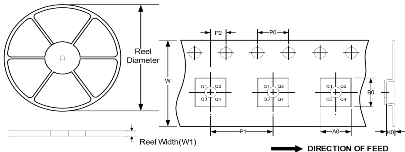
图 7. 包装编带尺寸
