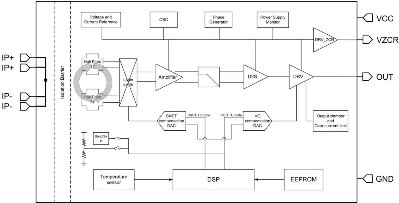
图.1 功能框图
