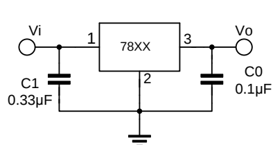
FIG.1 DC PARAMETERS
