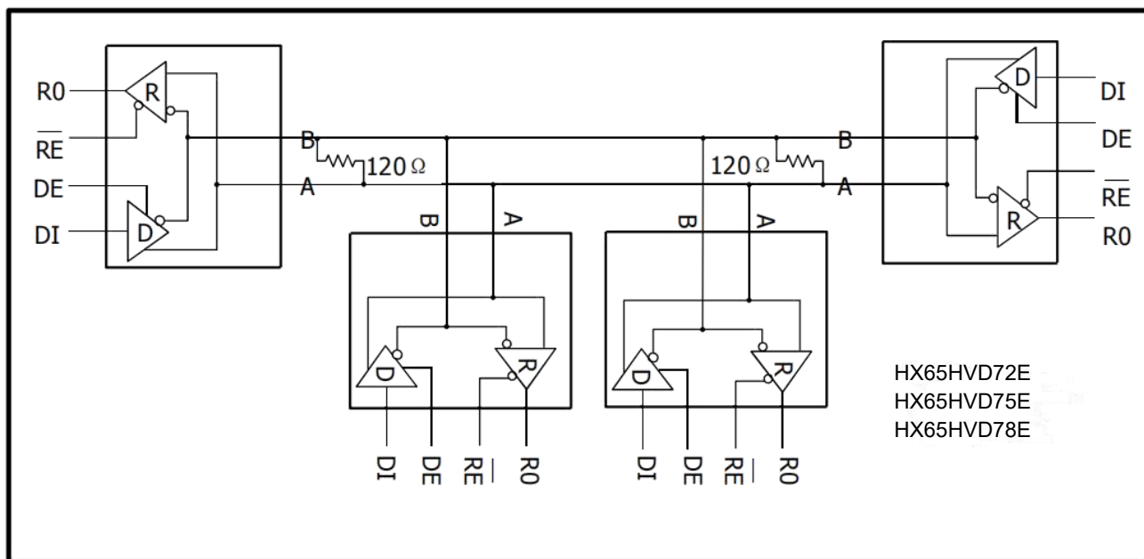
图 11. 典型半双工模式下 RS485 网络
