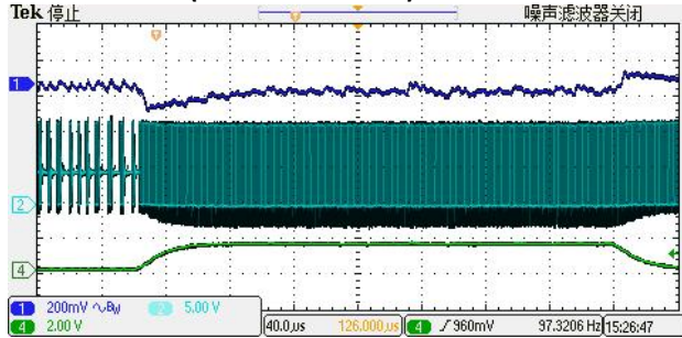
Load Transient(0.05A--1.5A Load)
