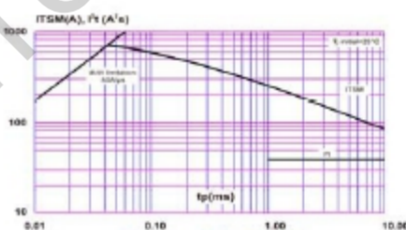
6、 I_{TSM}-I_1, I_2-t 曲线
