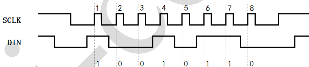
图 2 单字节通信
