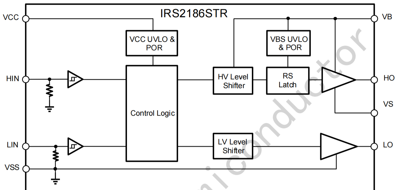
图7-4 IRS2186S功能框图
