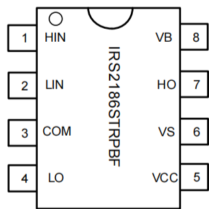
图 4-1 8-脚SOIC顶视图
