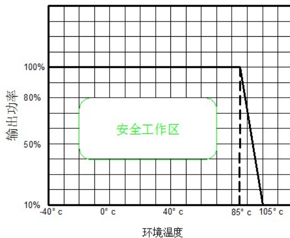
温度曲线图
