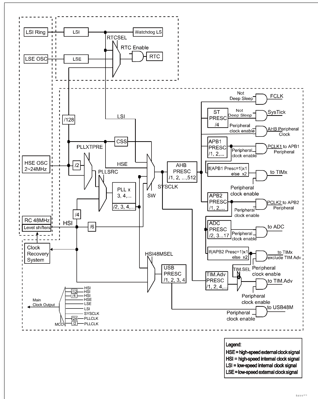
图 2-3 时钟树
