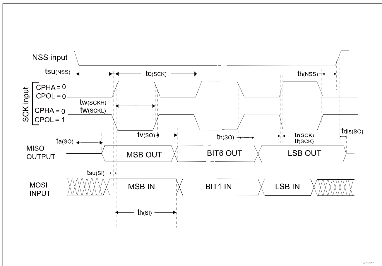
图 4-12 SPI 时序图-从模式和 CPHA = 0, CPOL = 1
