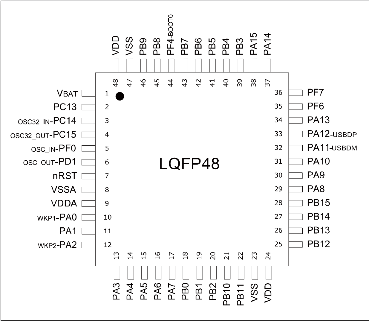
图 3-3 LQFP48 引脚分布
