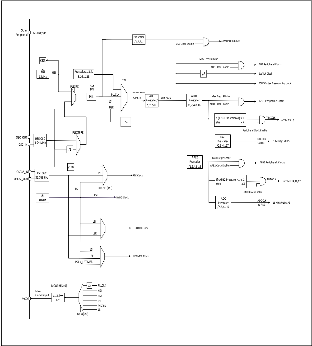
图 2-3 时钟树
