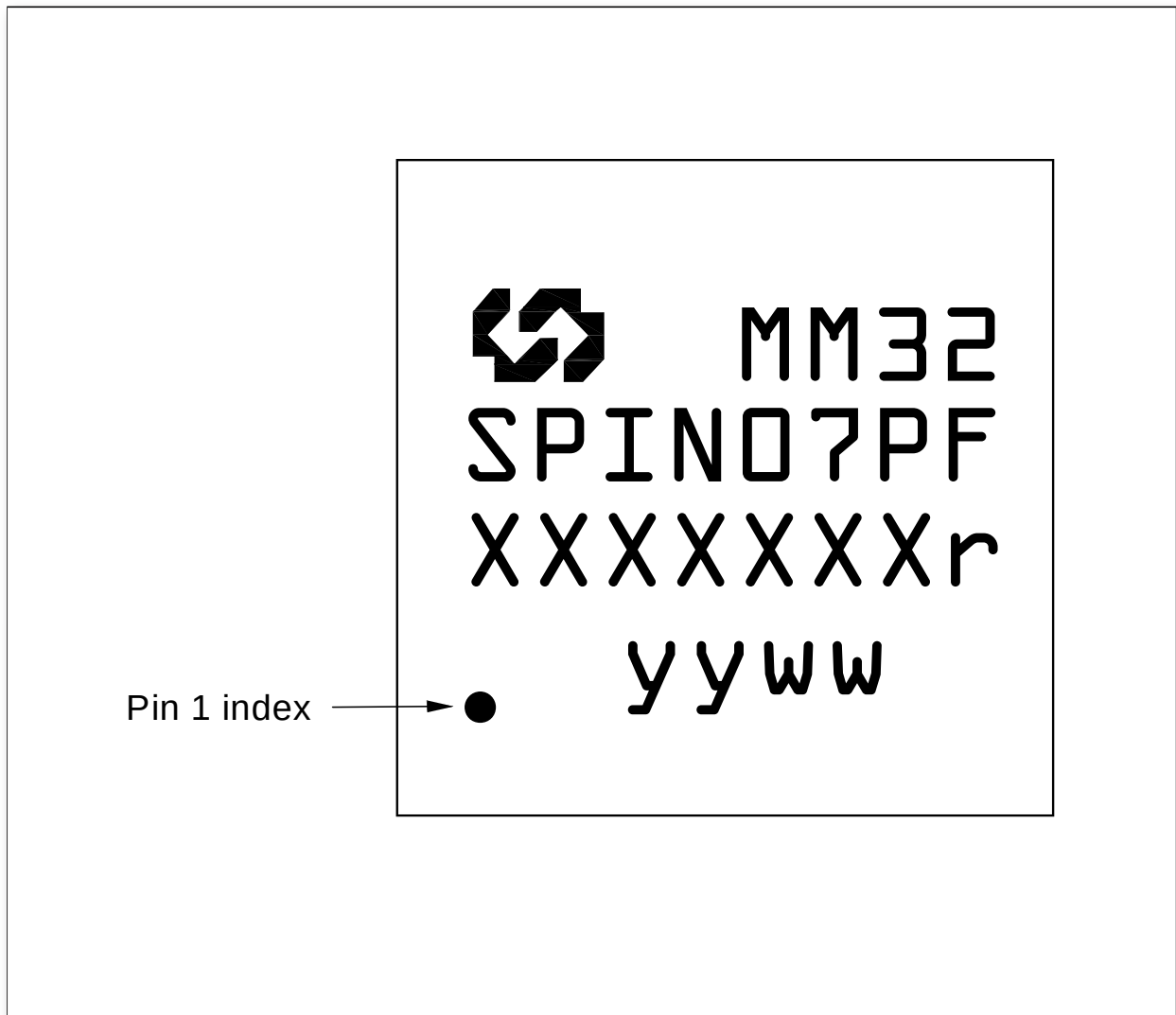
图 2-1 LQFP 和 QFN 封装丝印
