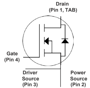
TO-247-4L (TO-247-4)
