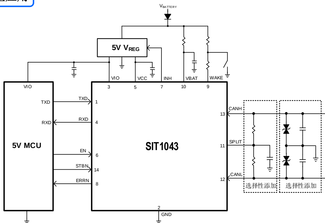
图 10 SIT1043 与 5V MCU 的典型应用图
