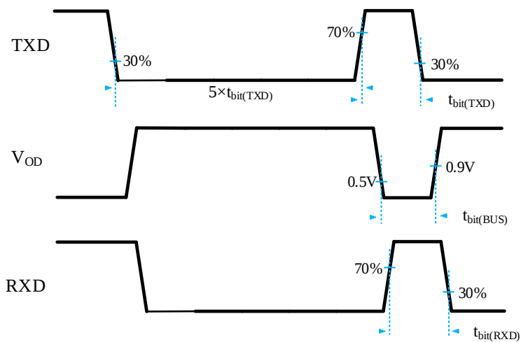
图 8 t_{bit} 延时示意图
