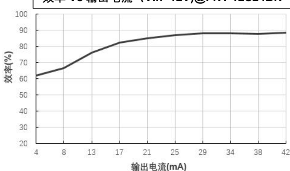
效率 Vs 输出电流 (Vin=12V)@FN1-12S24BN
