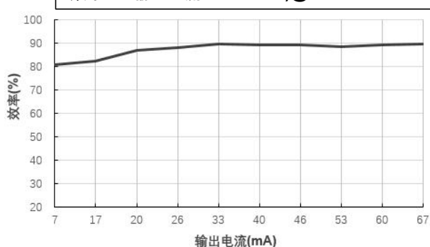
效率 Vs 输出电流 (Vin=12V)@FN1-12S15BN
