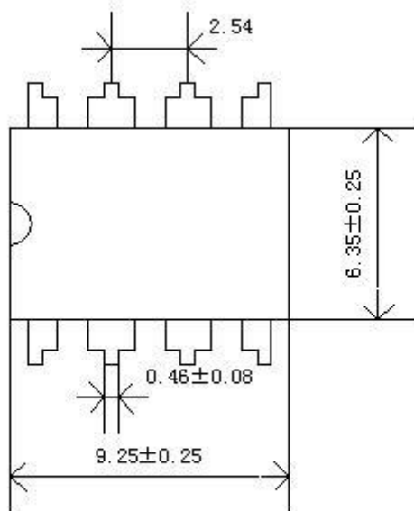
DIP8 封装尺寸
