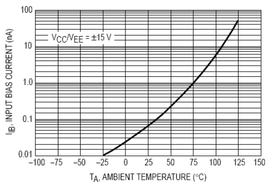
图3 输入偏置电流与温度的关系曲线
