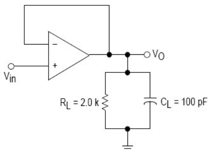
图1 单位增益电压跟随器
