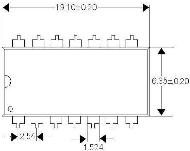
DIP14封装尺寸
