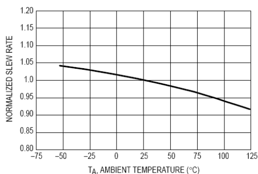
图11 标准的限摆率与温度的关系曲线
