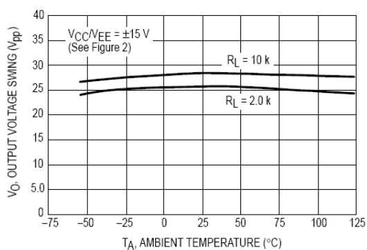
图7 输出电压摆动与温度的关系曲线
