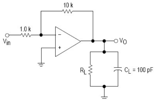
图2 反相放大器的增益为10
