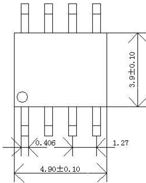
SOP8 封装尺寸
