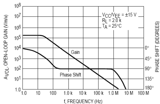
图9 大信号电压增益、相位位移与频率的关系曲线
