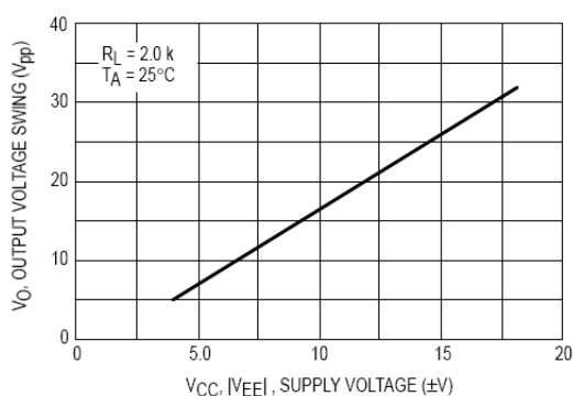
图6 输出电压摆动与供电电压的关系曲线
