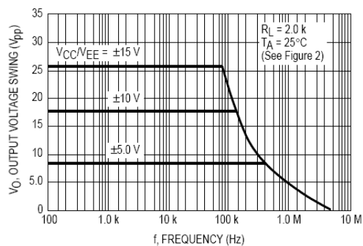
图4 输出电压摆动与频率的关系曲线
