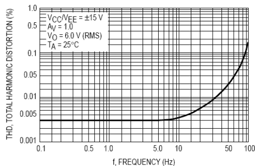
图13 总谐波失真与频率的关系曲线
