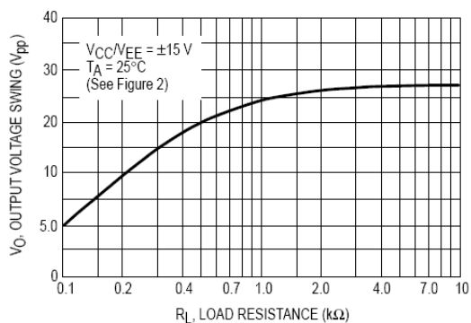
图5 输出电压摆动与负载电阻的关系曲线
