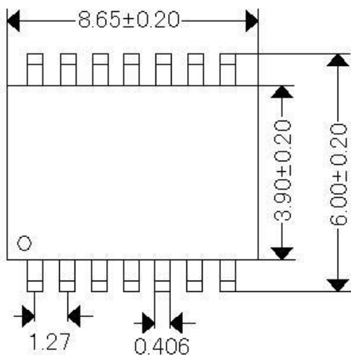
SOP14 封装尺寸
