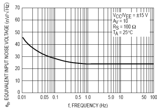
图12 等效输入噪声电压与频率的关系曲线
