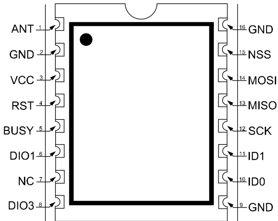
图 3-1 俯视图
